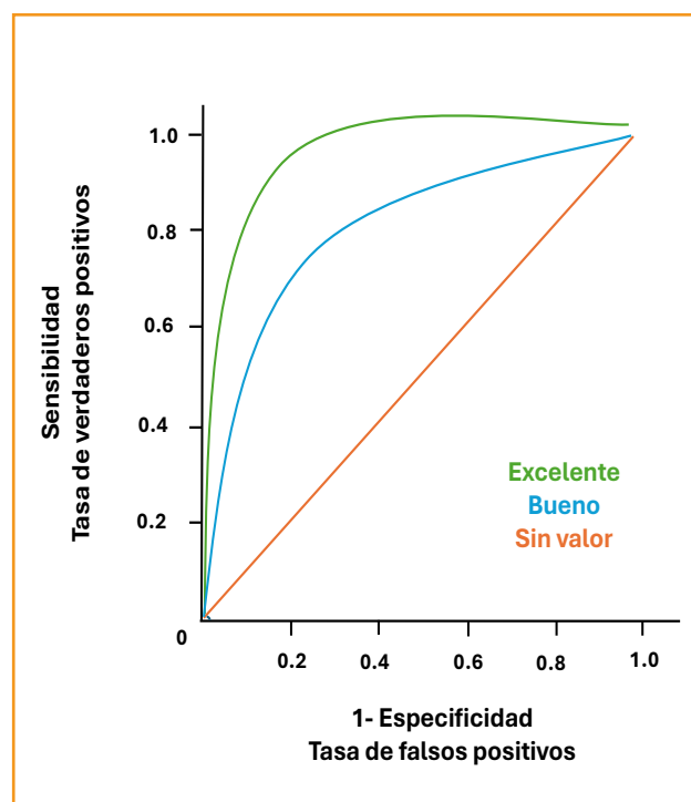
Figura 17. Ejemplo de curva ROC
